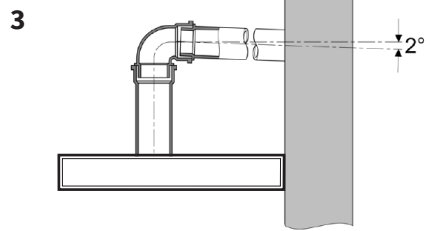
Abb. 3: Neigungswinkel der Abluftleitung
